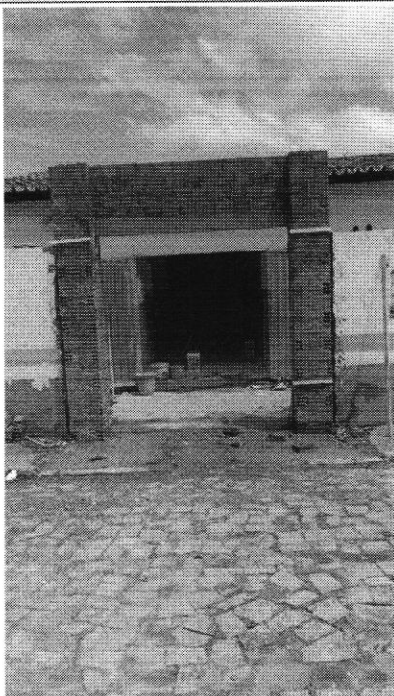
EXECUÇÃO DE ALVENARIA - UBS GATO
